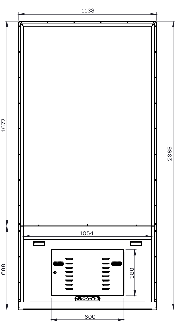
СХЕМА ДИСПЛЕЯ (ВИД СЗАДИ)
